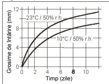
Diagrama 1: Viteza de întărire pentru SikaTack®-MOVE Transportation
