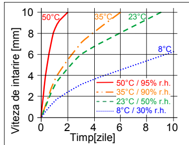
Fig 1: Viteza de intarire a sigilantilor Sikasil® monocomponenti
