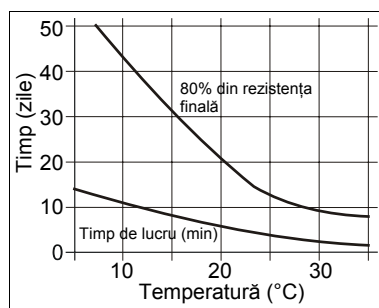
Diagramă: Timp de lucru și viteză de întărire pentru SikaFast®-5215
