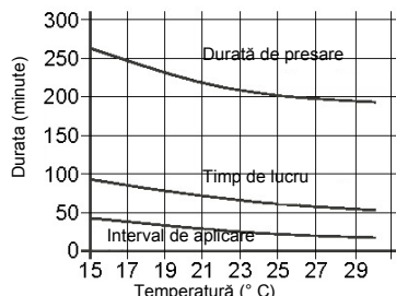
Figura 1: Durata de presare, timpul de lucru și intervalul de aplicare pentru SikaForce-7718 L30
