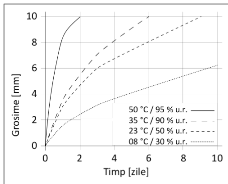
Diagrama 1: Viteza de întărire pentru Sikasil® AS-70
