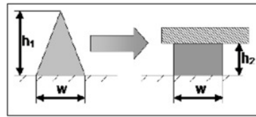
Figura 1. Dimensiunea recomandata a cordonului de adeziv
